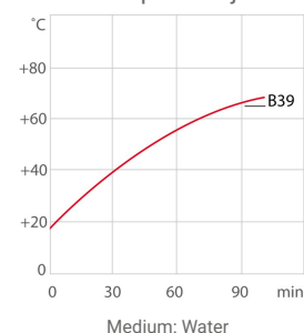
Opwarmtijd
