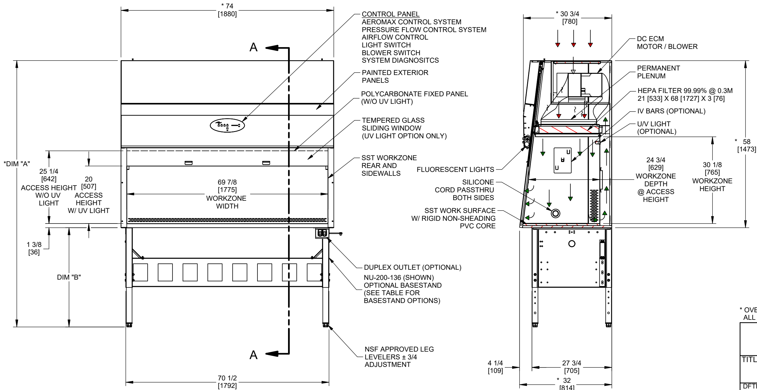
SECTION A-A
