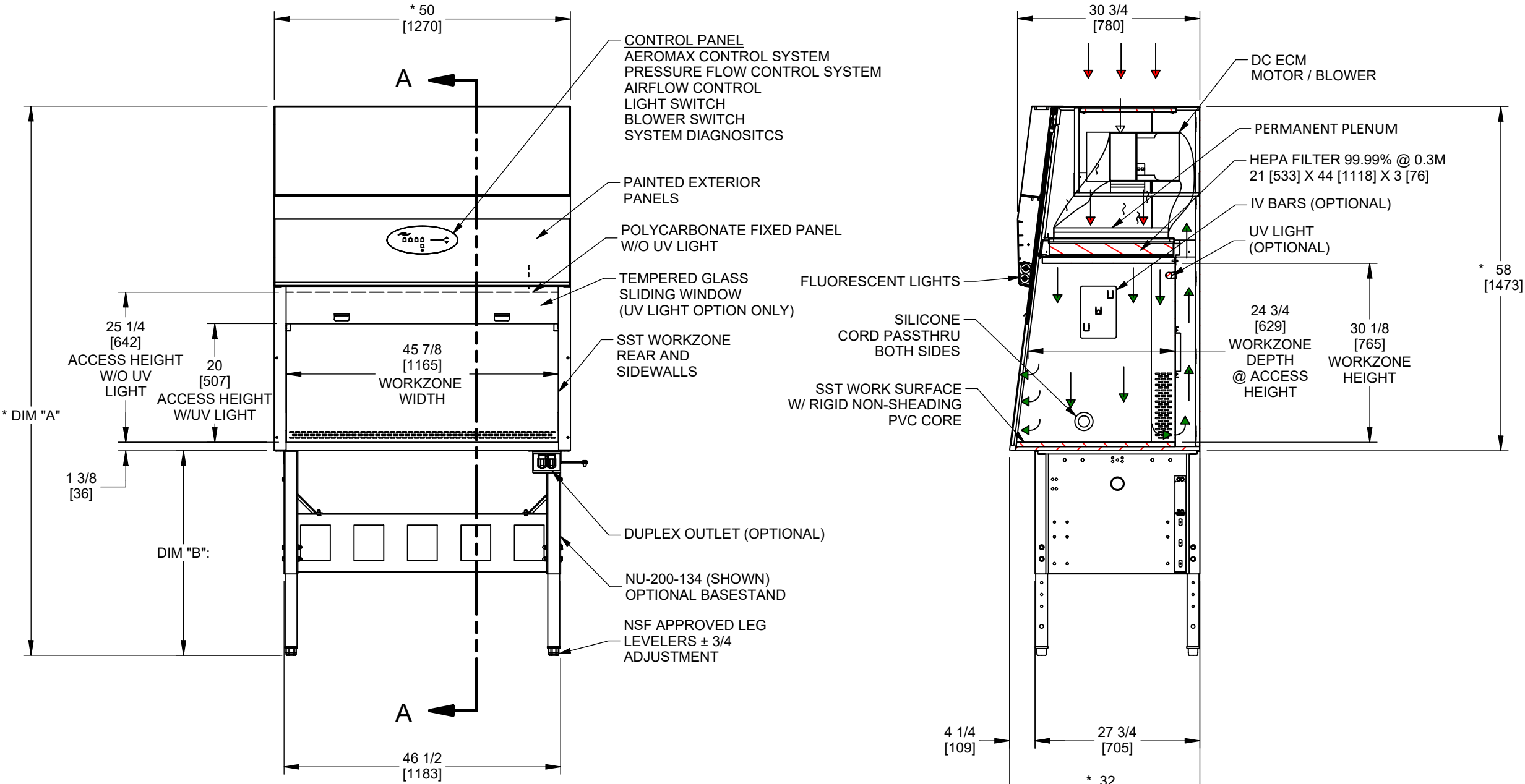
SECTION A-A
