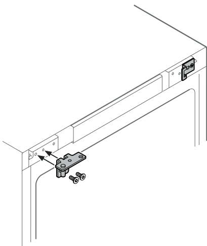
21. Scharnierbeugel vastschroeven.
