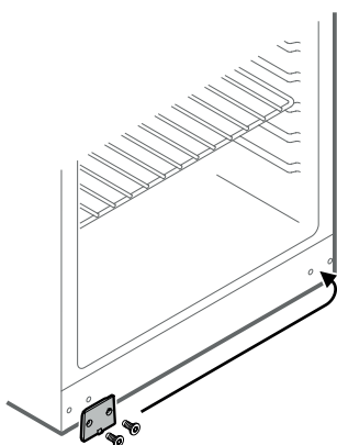
21. Scharnierbeugel vastschroeven.
