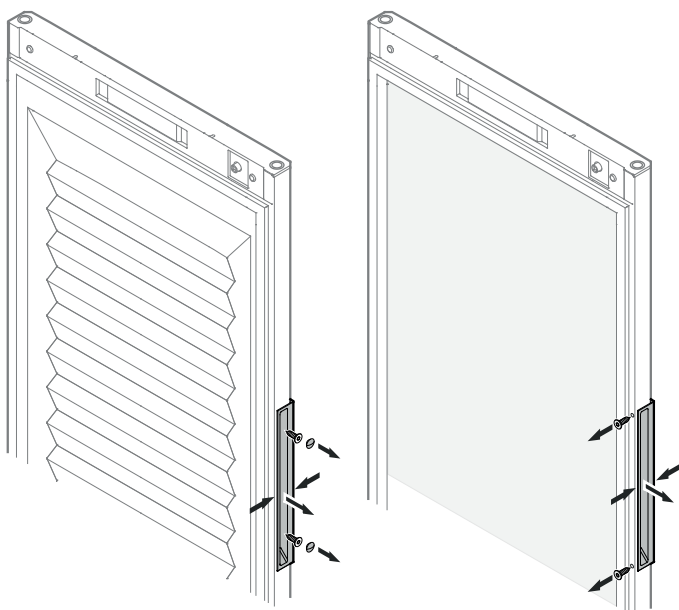
25. Greep vastschroeven.
