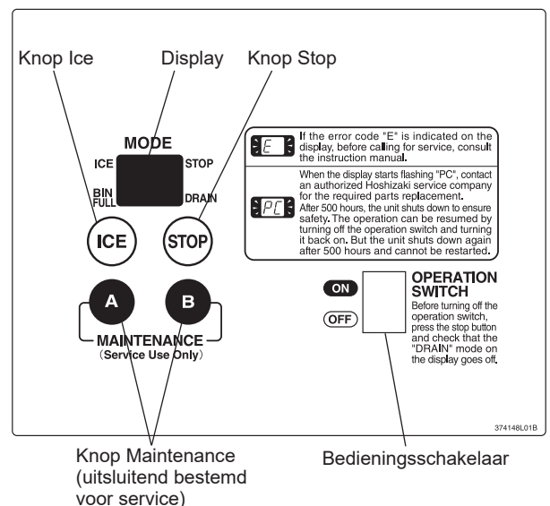
Bedieningspaneel
