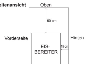
Seitenansicht
