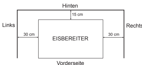
Ansicht von oben (nur FM-600AKE)
