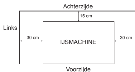
Bovenaanzicht (uitsluitend FM-600AKE)
