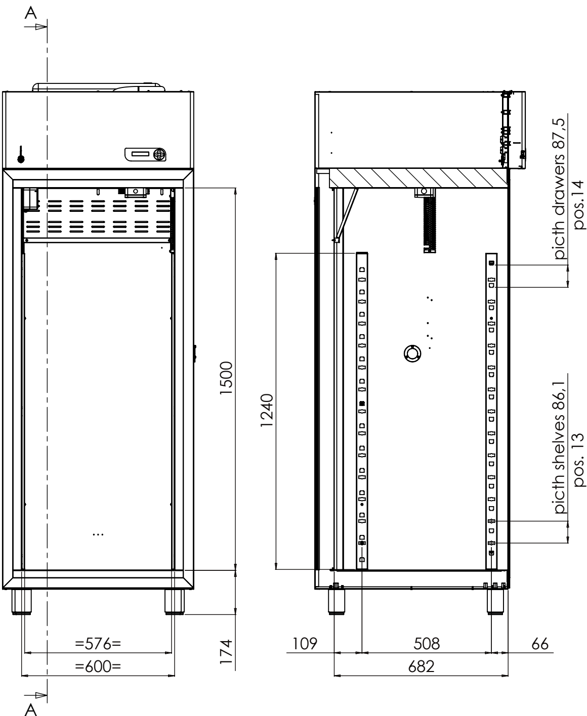
SECTION A-A
