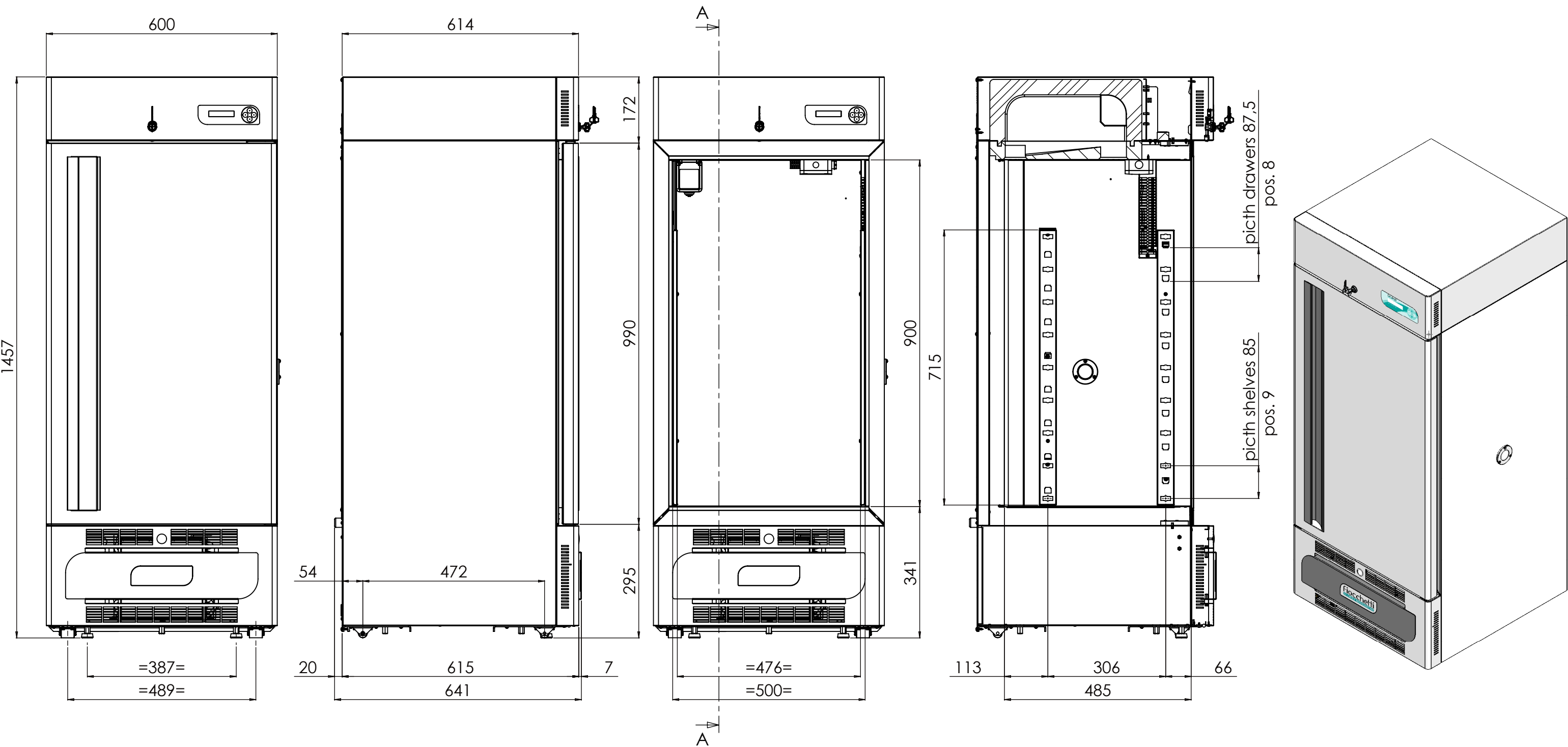
SECTION A-A
