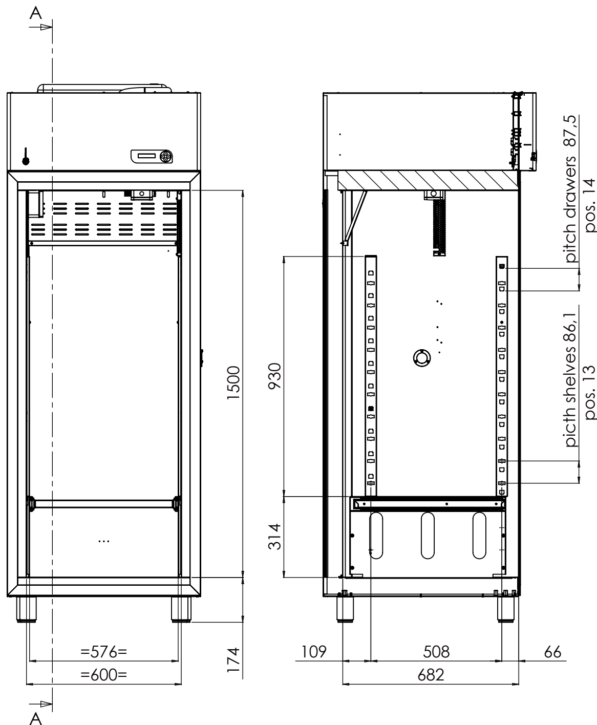
SECTION A-A
